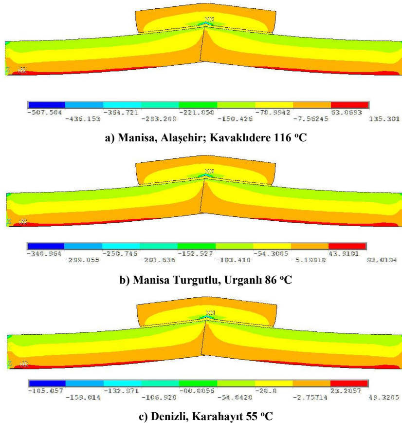
Şekil 5: Tüm model üzerinde \sigma_x normal gerilmeleri
