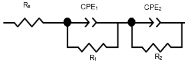
Şekil 7: Eşdeğer elektrik devre şeması
