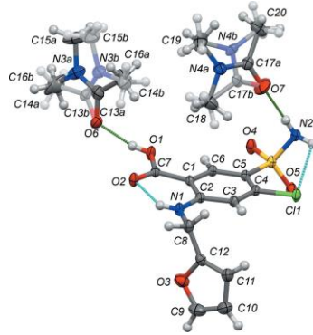
Şekil 12: Beloborodova ve arkadaşlarının sentezlediği co-kristal yapısı
