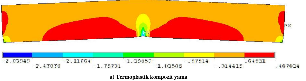
Şekil 11: Kompozit yama üzerinde \sigma_x normal gerilmeleri
