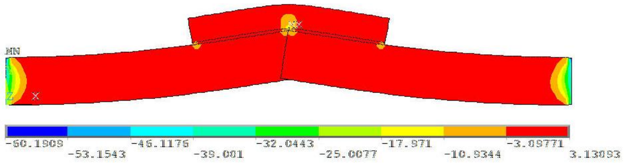
Şekil 6: Tüm model üzerinde \sigma_y normal gerilmeleri
