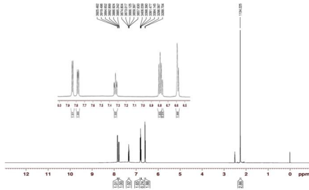
EK 7 (H 2 a4mp)(salic) Bileşiğinin 1 H-NMR spektrumu
