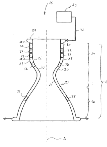
Şekil 10: US20180143126 numaralı patent başvurusunda bahsedilen roket motor gövdesi
