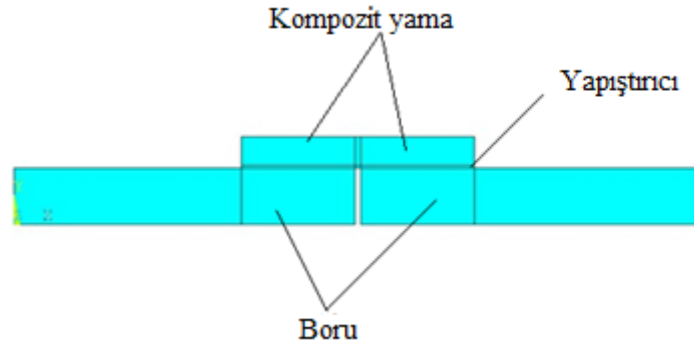
Şekil 12: Katı model
