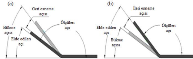
Şekil 2: Bükmede geri ve ileri esneme davranışları; a) geri esneme, b) ileri esneme [11]
