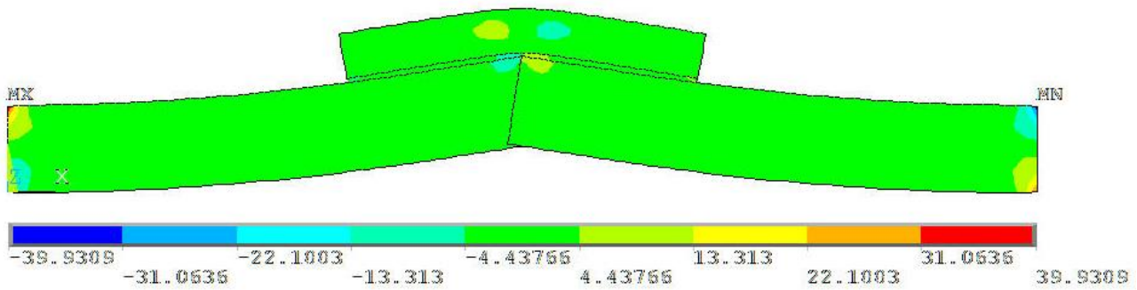
Şekil 7: Tüm model üzerinde \tau_{xy} kayma gerilmeleri
