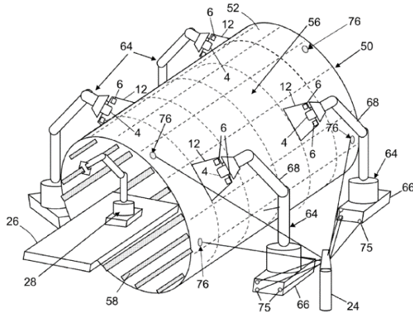
Şekil 6: US9519844 Patent Dokümanında Geçen Kızılötesi Termografik Muayene Sistemi [7]
