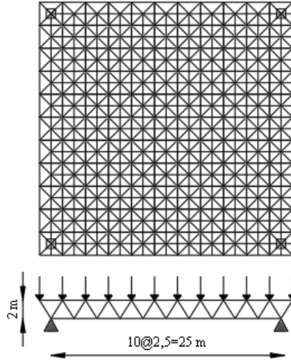
Şekil 7: Çift katmanlı uzak kafes sistem geometrisi
