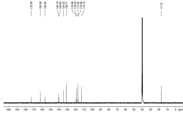
EK 6 (H 2 a3mp)(salic) Bileşiğinin 13 C-NMR spektrumu
