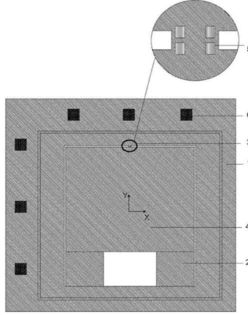
Şekil 4: CN104391133B numaralı patentte geçen MEMS sensor [7]
