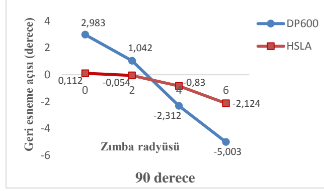
Şekil 4: Kalıp açısı ve zımba radyüsü etkisinde oluşan geri esneme grafikleri; a) 30, b) 60, c) 90 derece kalıp açısı
