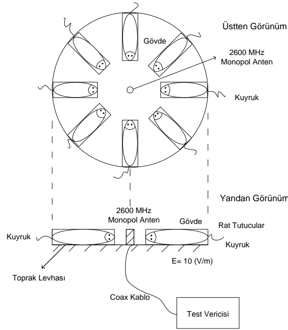
Şekil 2: Deney düzeneği
