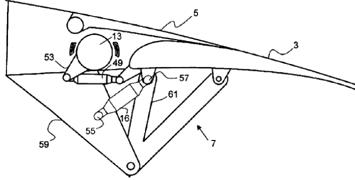
Şekil 8: US9573676B2 numaralı patente geçen ayarlanabilir flap için cihaz
