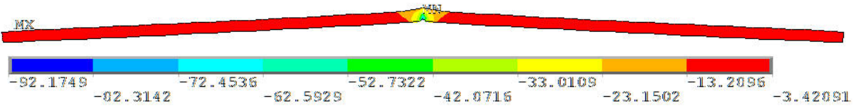
Şekil 8: Yapıştırıcı tabaka üzerinde \sigma_x normal gerilmeleri
