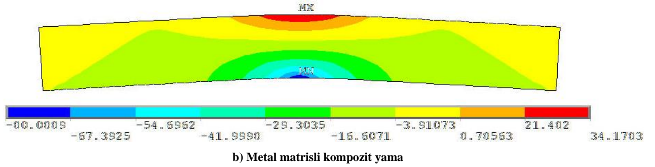
Şekil 11: Kompozit yama üzerinde \sigma_x normal gerilmeleri
