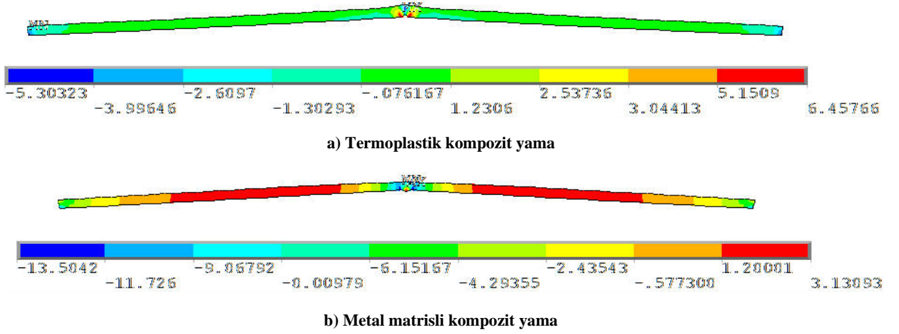
Şekil 9: Yapıştırıcı tabaka üzerinde \sigma_y normal gerilmeleri
