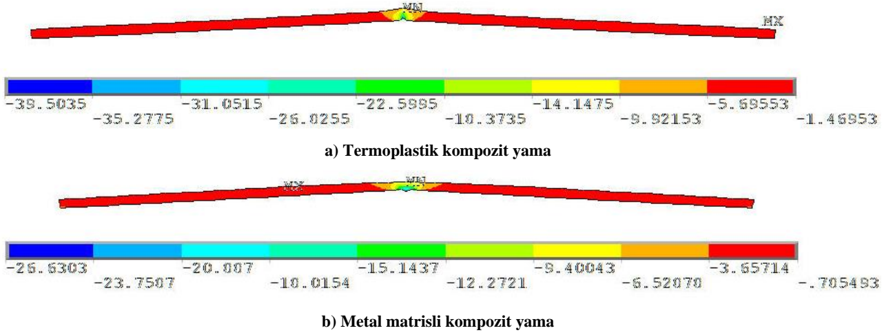
Şekil 8: Yapıştırıcı tabaka üzerinde \sigma_x normal gerilmeleri
