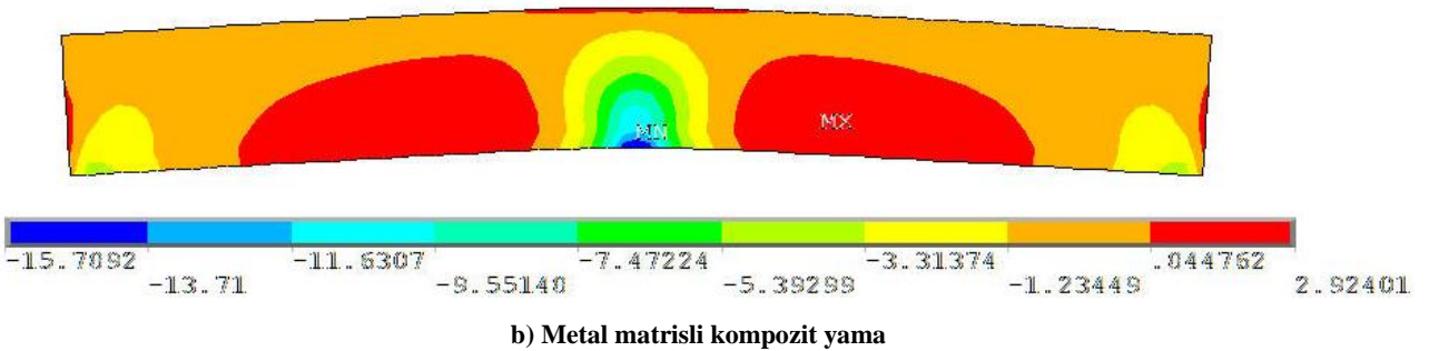
Şekil 12: Kompozit yama üzerinde \sigma_y normal gerilmeleri
