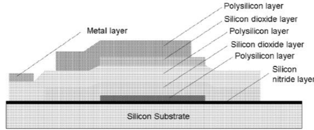
Şekil 5: US20110138902A1 numaralı patentte geçen MEMS cihazının üretim aşaması [8]
