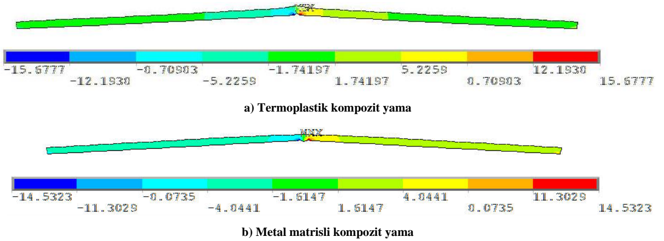
Şekil 10: Yapıştırıcı tabaka üzerinde \tau_{xy} kayma gerilmeleri
