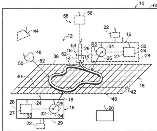
Şekil 5: US20180154588 numaralı patentte ek kürlenme kaynağı
