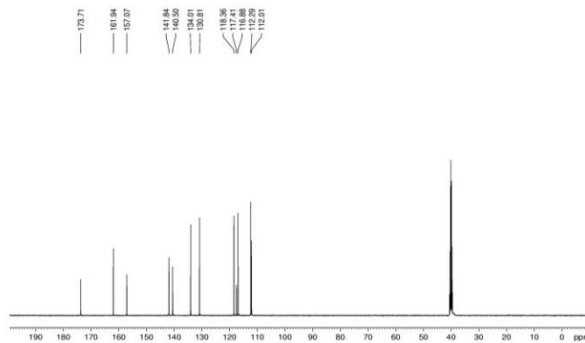
EK 3 (H 2 ap)(salic).0,01EtOH Bileşiğinin 13 C-NMR spektrumu
