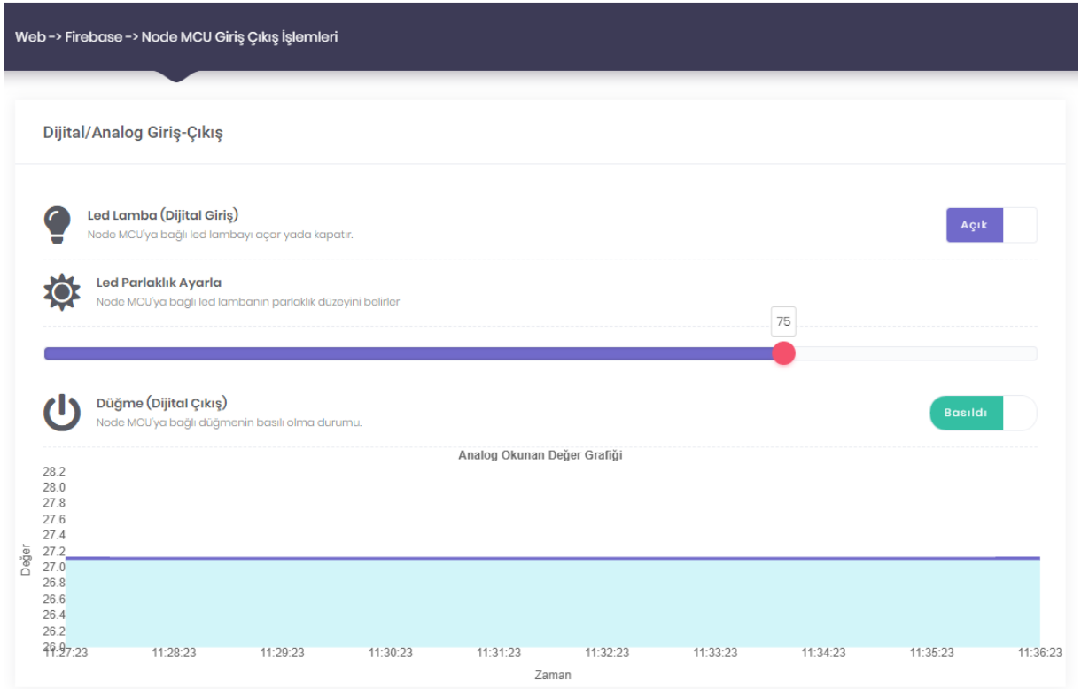
Şekil 29: Web arayüzü
