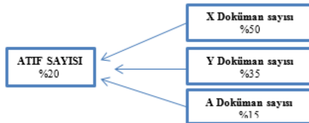
Şekil 4: Atf Sayısı
