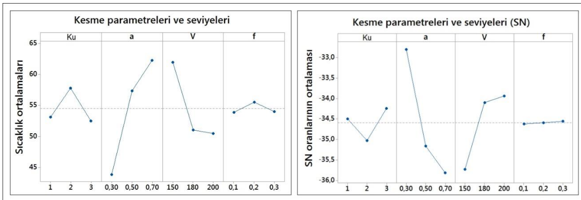
Şekil 3. Kesme parametrelerinin seviyeleri için etki grafikleri
