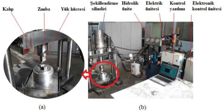
Şekil 1: Deney düzeneğinin genel görünümü; a) detay görünüm, b) genel görünüm
