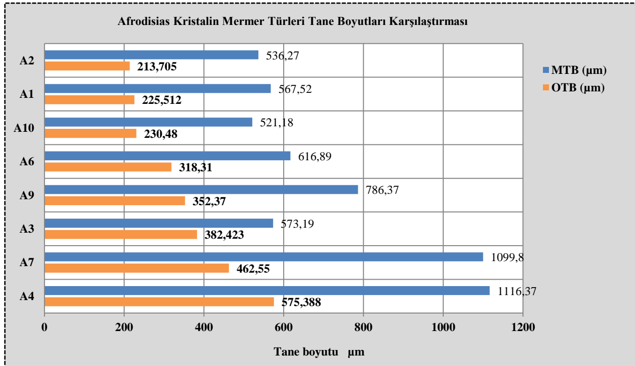
Şekil 10: Afrodiasias kristalin mermerlerin Ortalama tane boyutu (OTB) ve maksimum tane boyutu (MTB) karşılaştırma grafiği. A: Afrodiasias kristalin mermer türleri.
