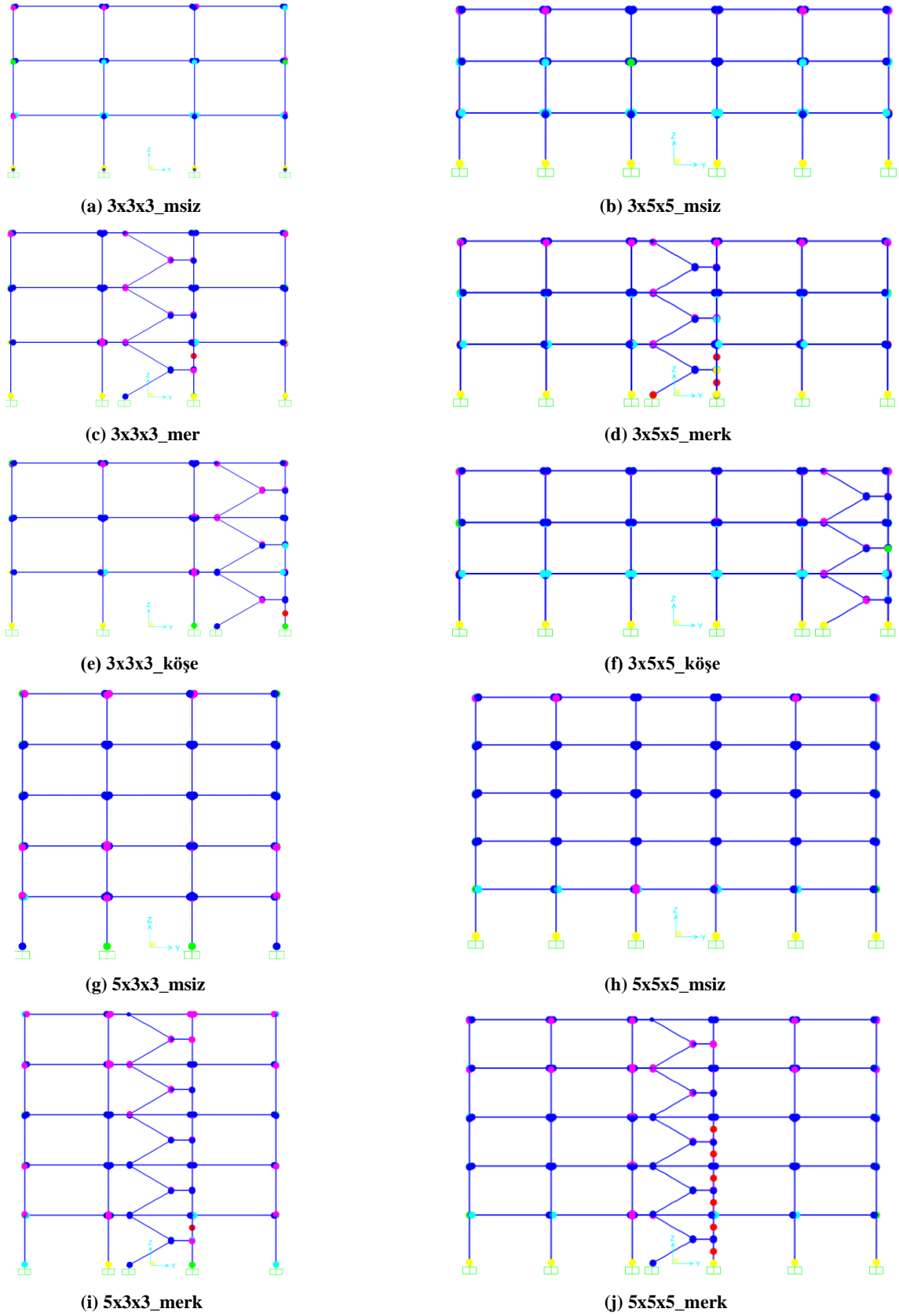
Şekil 8: Modellerin Plastik Mafsıl Dağılımları
