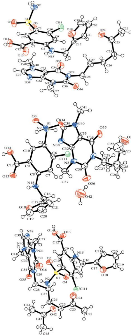
Şekil 17: Stepanovs ve Mishnev'in sentezlediği co-kristal yapıları
