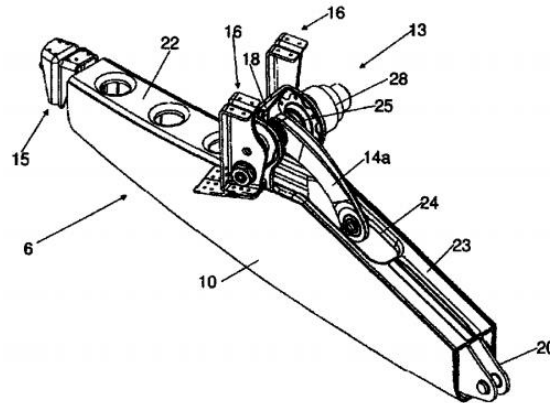
Şekil 10: CN103029827A numaralı patente geçen flap destek elemanı
