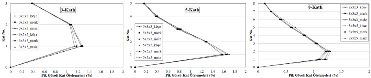
Şekil 3: Katlarda meydana gelen ortalama pik görel kat ötelemeleri
