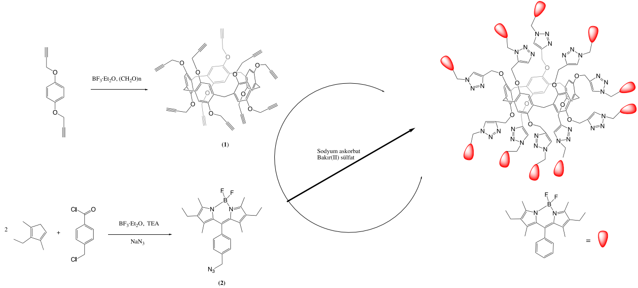
Şema 1 Hedef bileşiğin reaksiyon rotası.
