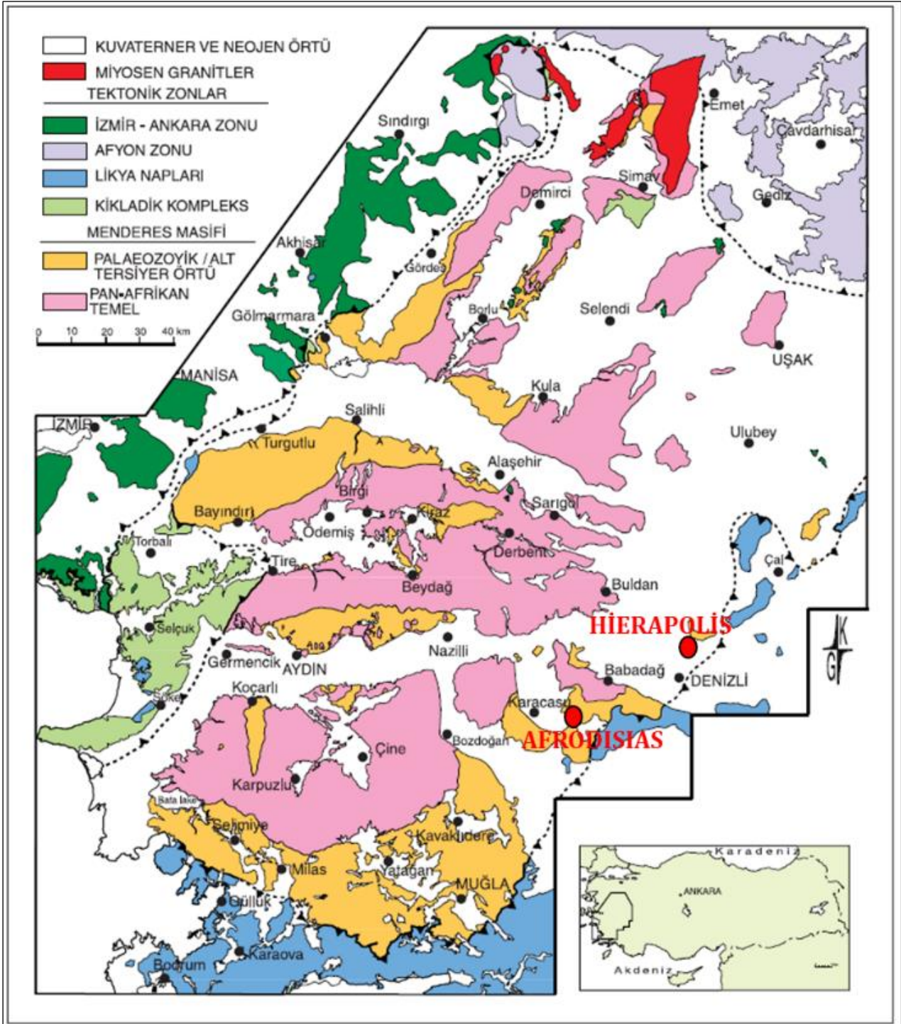
Şekil 5: Menderes Masifinin bölgesel jeolojik yapı içindeki genelleştirilmiş jeolojik haritası (Candan ve diğ. 2011), Afrodisias ve Hierapolis antik kentlerinin yeri.
