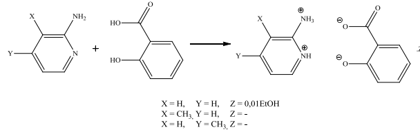
Şekil 1: Proton transfer tuzlarının sentezi
