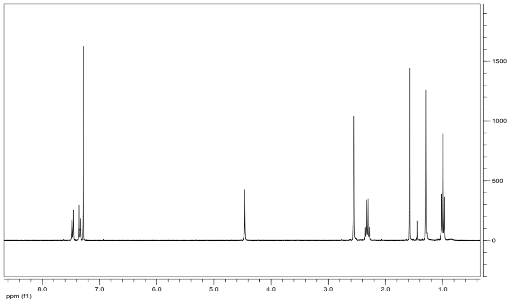
Şekil 2 Bileşik 2'nin ^1\text{H-NMR} spektrumu
