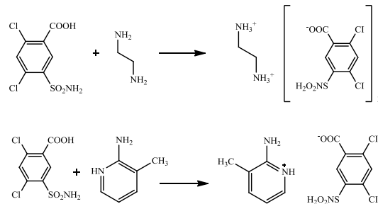
Şekil 11: Yenikaya ve arkadaşlarının sentezlediği proton transfer tuzları
