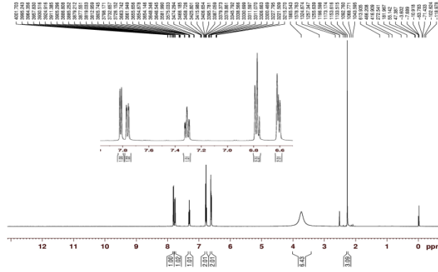
EK 8 (H 2 a4mp)(salic) Bileşiğinin D 2 O ilaveli 1 H-NMR spektrumu
