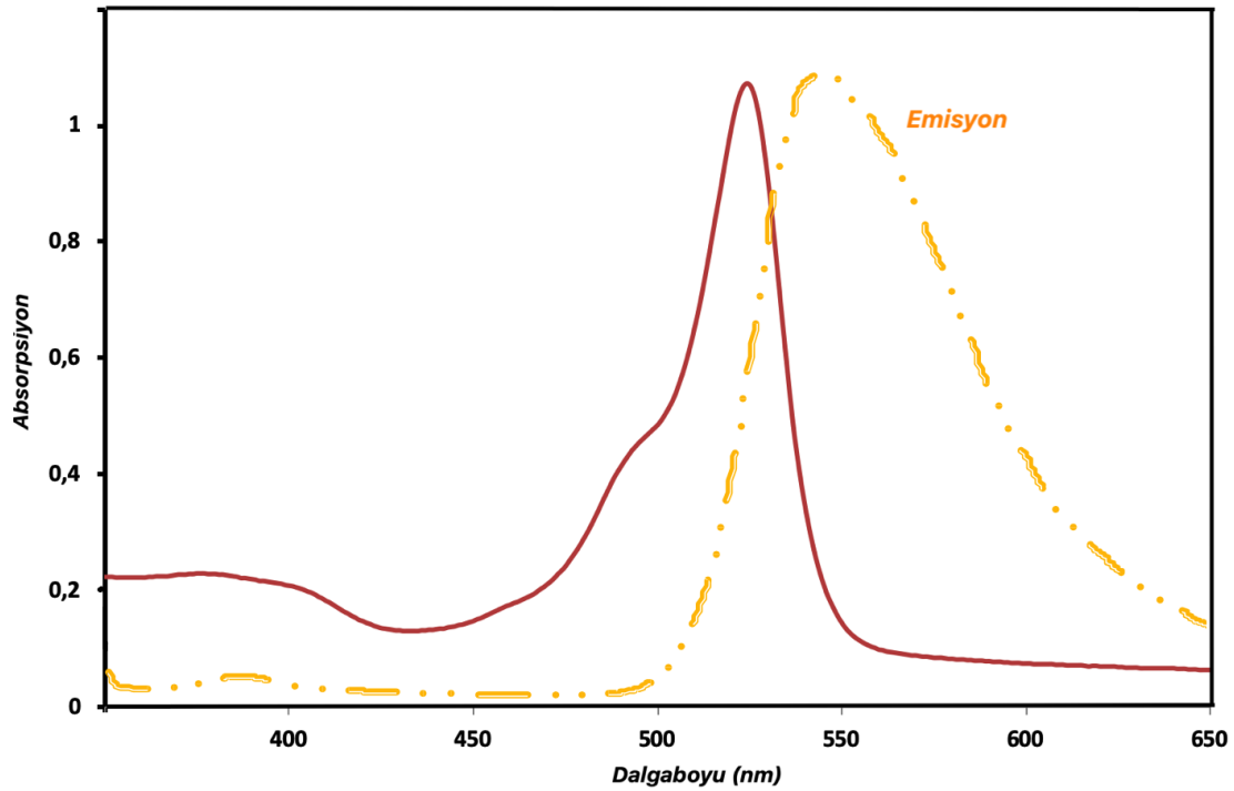
Şekil 3 Bodipy temelli pillar[5]aren bileşiğinin normalize edilmiş absorpsiyon ve emisyon spektrumları
