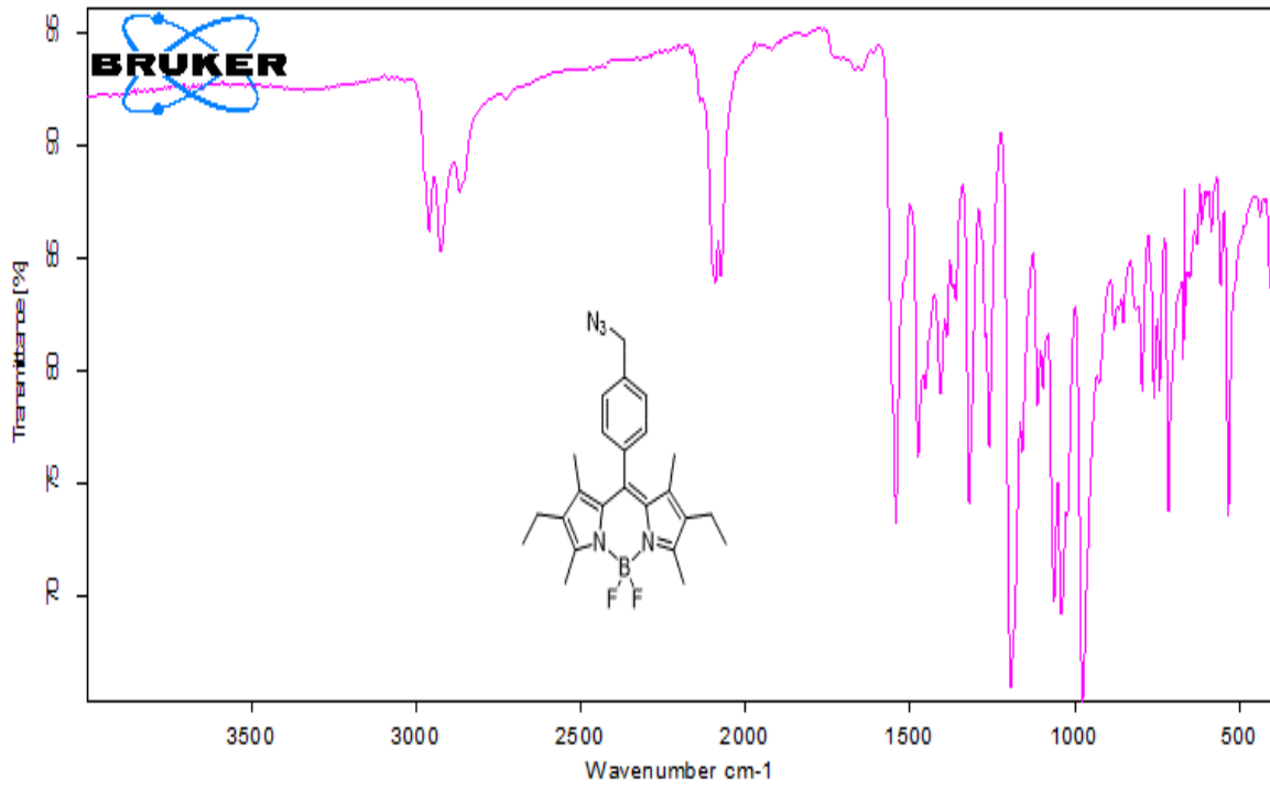
Şekil 1 Bileşik 2'nin FT-IR spektrumu
