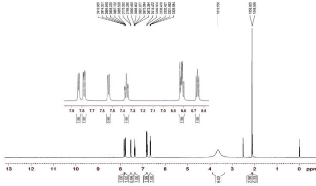
EK 5 (H 2 a3mp)(salic) Bileşiğinin D 2 O ilaveli 1 H-NMR spektrumu
