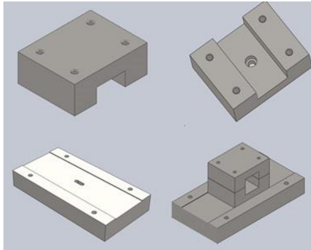
Şekil 2: Solidworks ile tutucu parçaların tasarlanması
