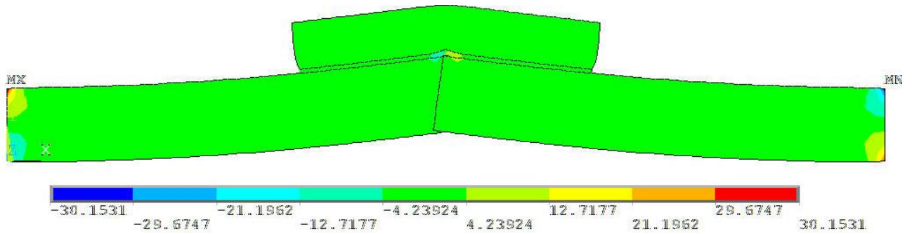
Şekil 6: Tüm model üzerinde \sigma_y normal gerilmeleri
