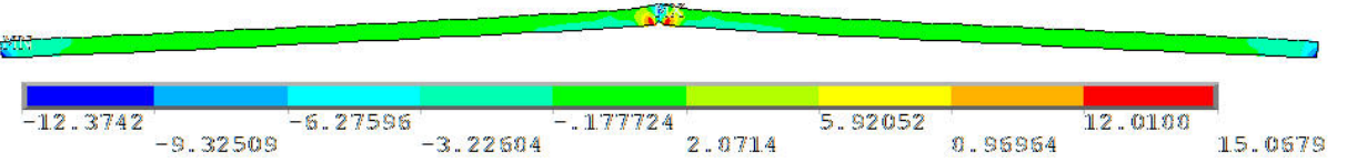
Şekil 9: Yapıştırıcı tabaka üzerinde \sigma_y normal gerilmeleri
