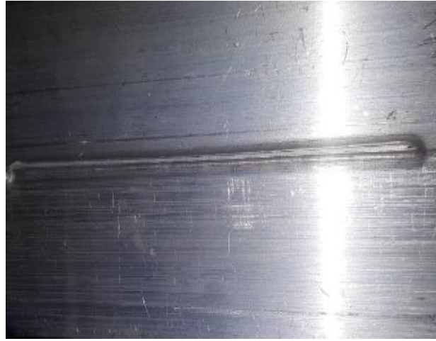
Şekil 4: Kaynak sonrası arka dikiş görünümü
